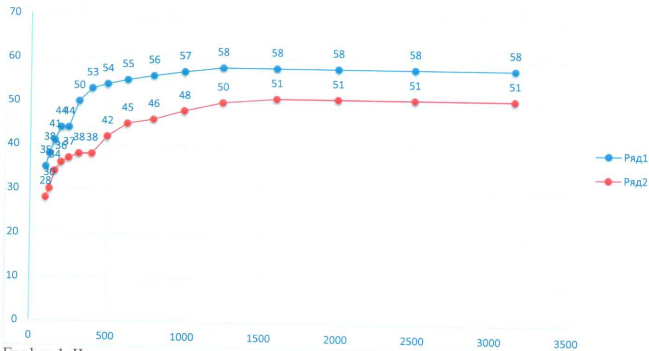
График 1. Частотная характеристика изоляции воздушного шума, Где,
